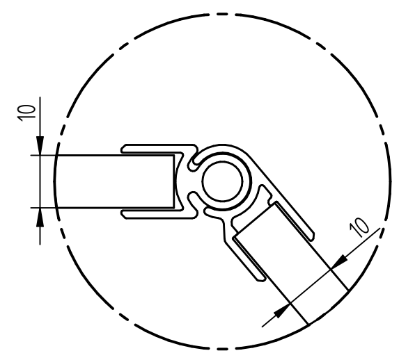
EINZELHEIT A
